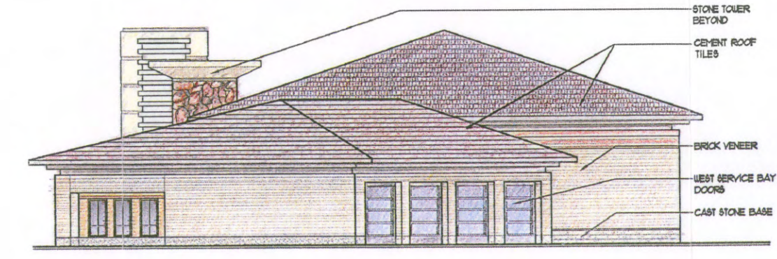
5 NORTH ELEVATION SCALE: 1/8" = 1'-0"
