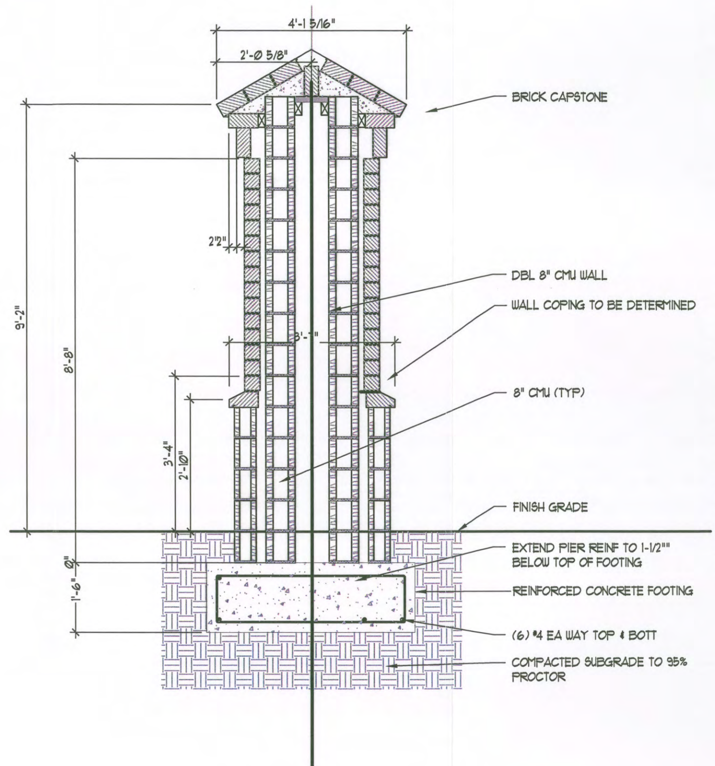
2 SECT THRU PILASTER AI-01 SCALE: 1/2" = 1'-0"
